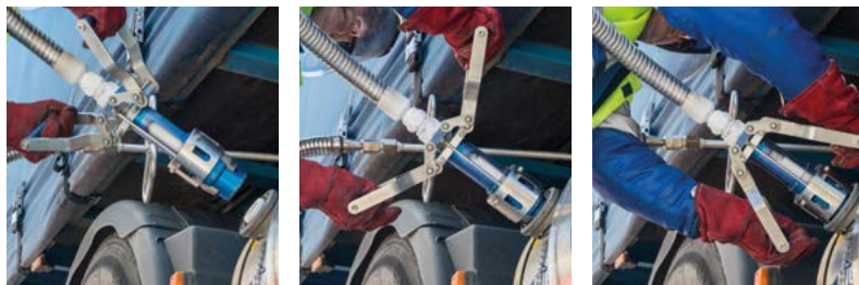
Detalle de la conexión de la manguera de GNL al vehículo
